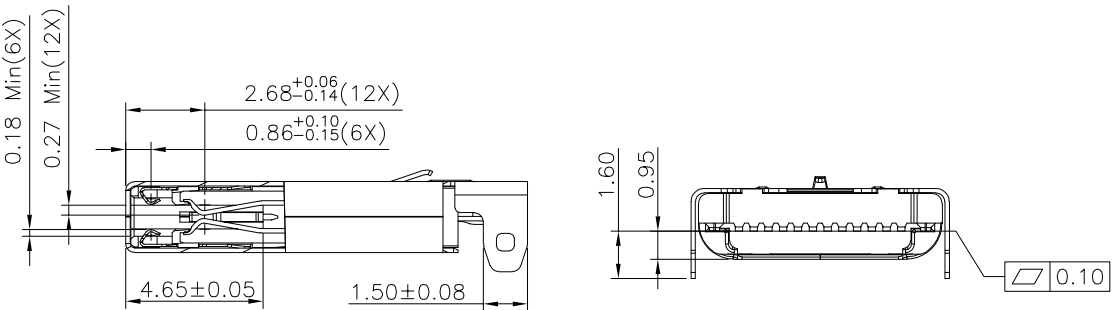
SECTION:A-A SCALE 1:1
