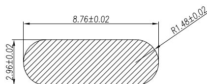
治具/外壳装硅胶圈位置尺寸示意图
