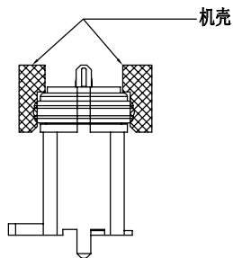
组装示意图
