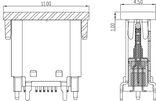
装吸取盖示意图
